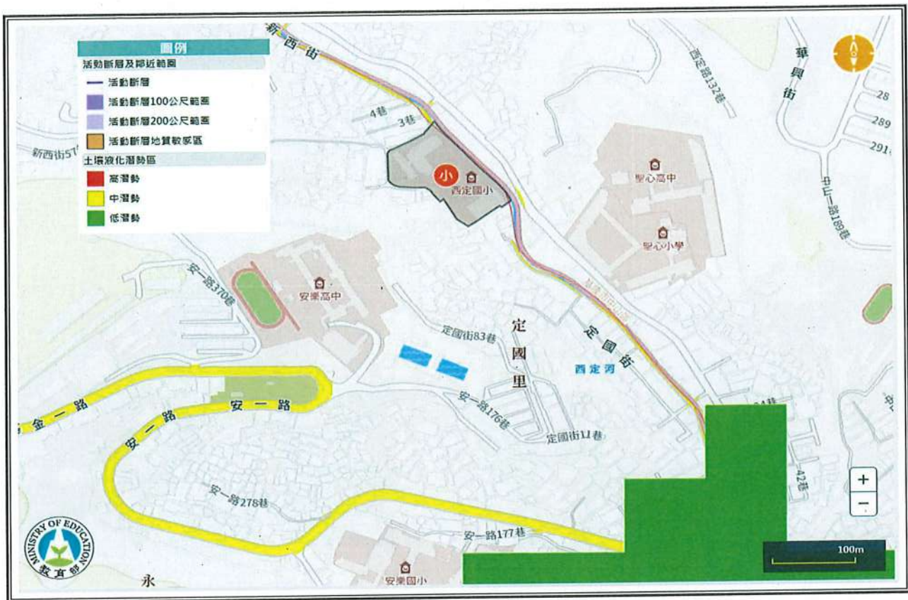
圖 2.4.1 地震災害潛勢圖 (瀏覽日期：115 年 9 月 7 日)
