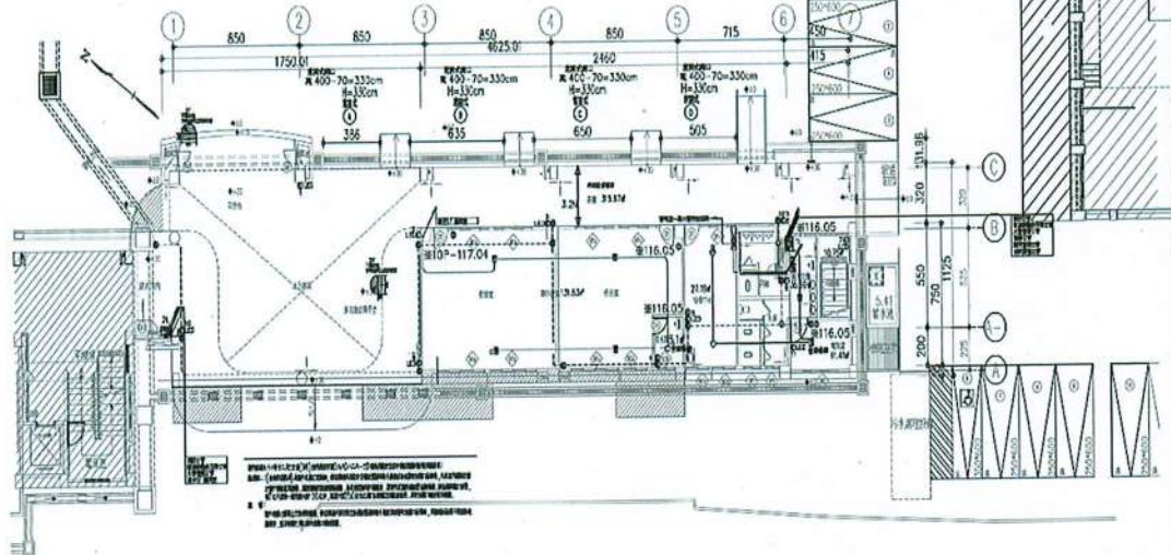
新善樓1F平面圖 5.1-100
