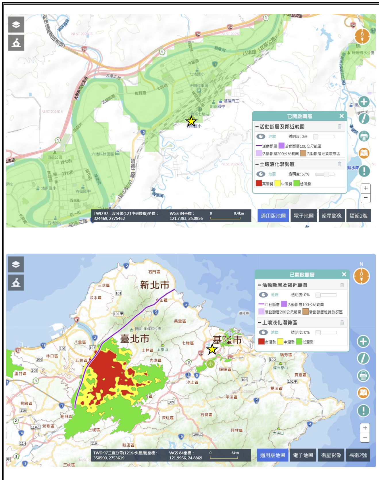
圖 2.4.1 地震災害潛勢圖 (瀏覽日期: 115 年 8 月 4 日)
