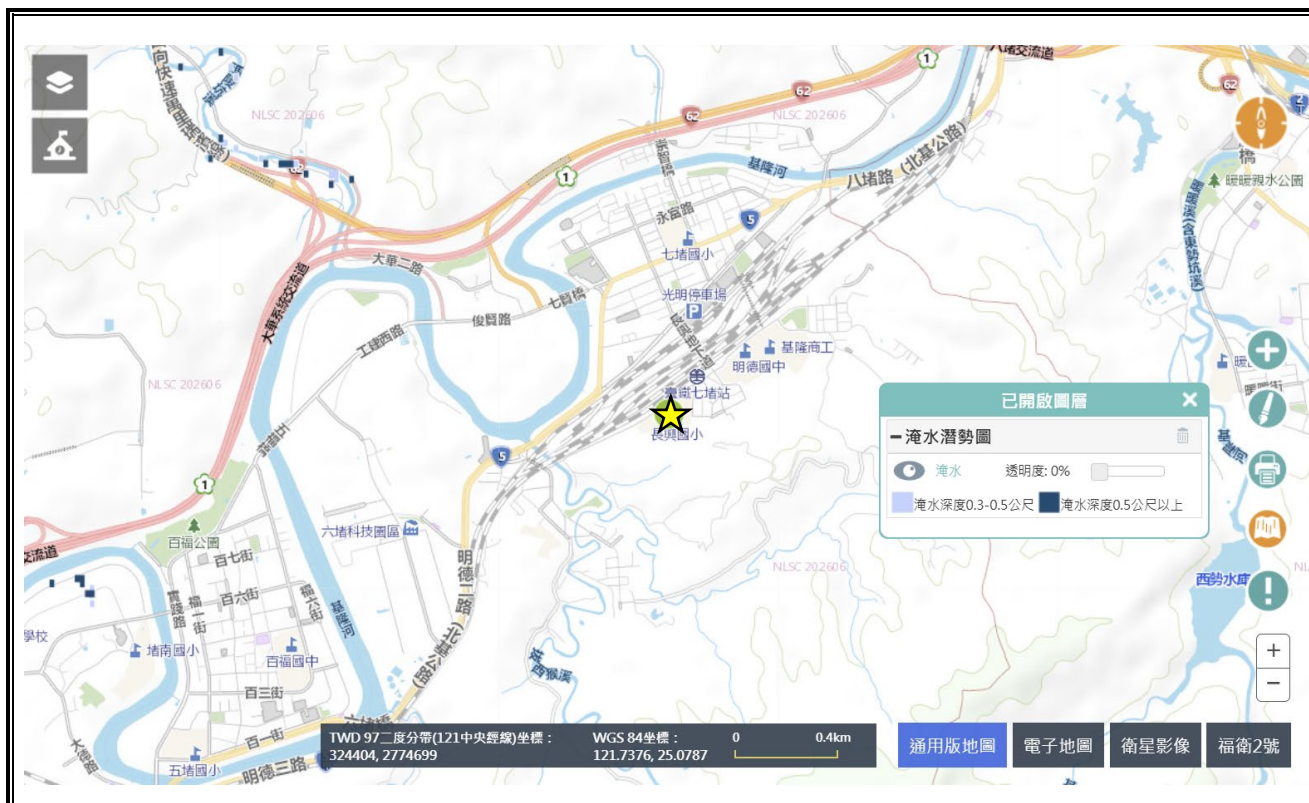
圖 2.4.2 淹水災害潛勢圖 (瀏覽日期： 115 年 8 月 4 日)
