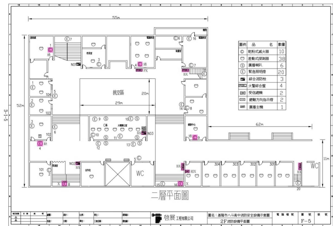
平面圖
