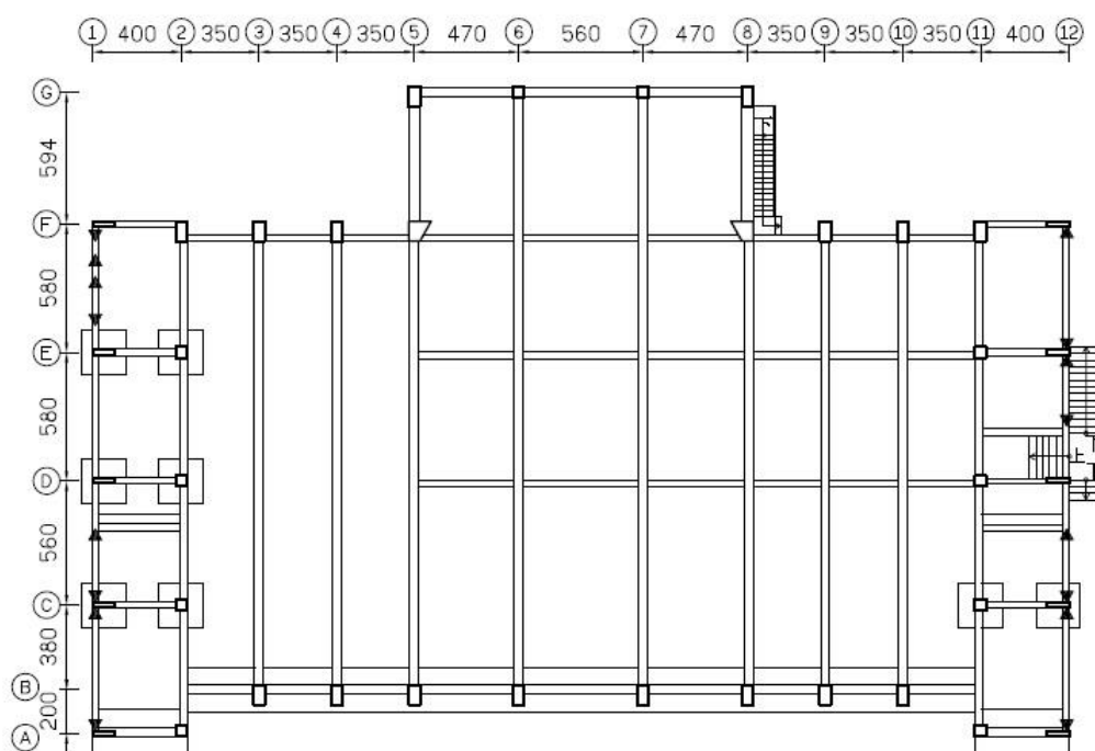
一樓結構平面圖 S=1/300 (方案一)
