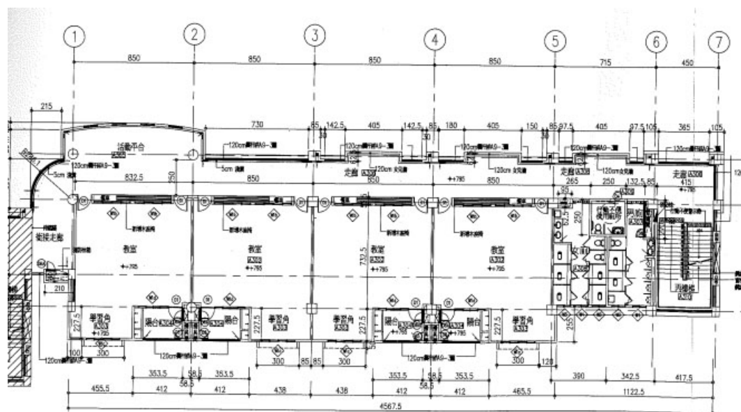
參層平面圖 S:1/100
