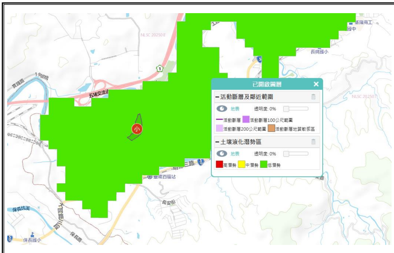
圖 2.4.1 地震災害潛勢圖 (瀏覽日期： 114 年 9 月 15 日)
